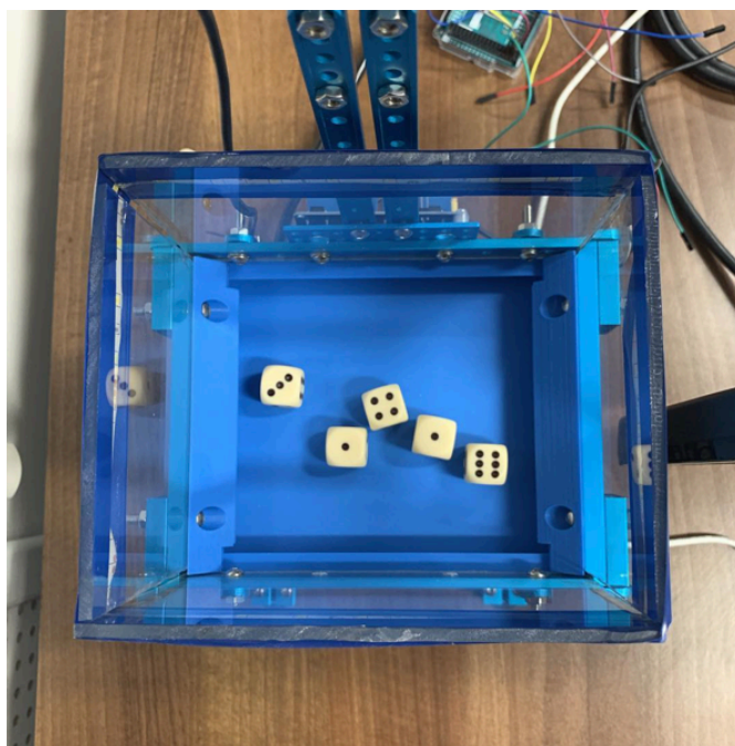
Kockovrh - stroj na automatické hádzanie kociek a detekciu hodených čísel pomocou kamery a algoritmov na spracovanie obrazu
